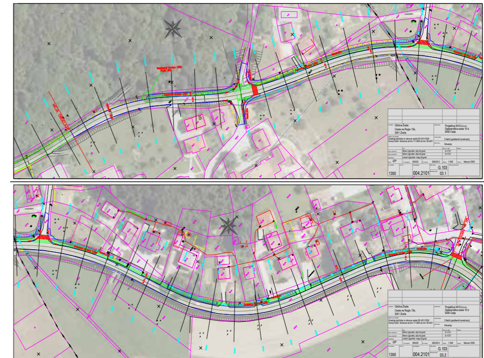
Predvidena rekonstrukcija ceste s pločnikom in kolesarsko stezo Stranice proti Vitanju
