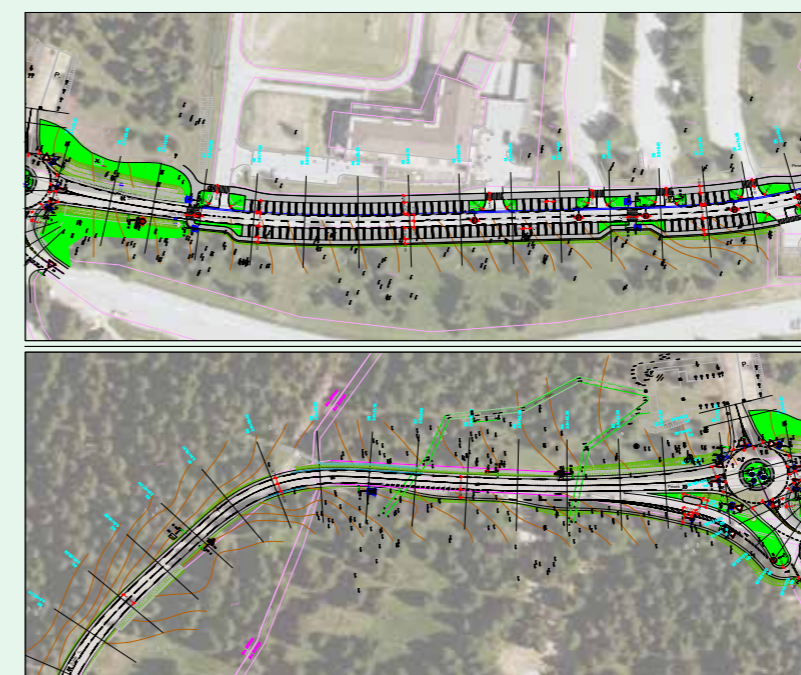
Predvidena rekonstrukcija ceste Zreče-Rogla, Regionalna cesta R3-701/1430, km 2+850–km 5.500 na Rogli
